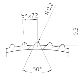
Детализация рёбер (10:1)
